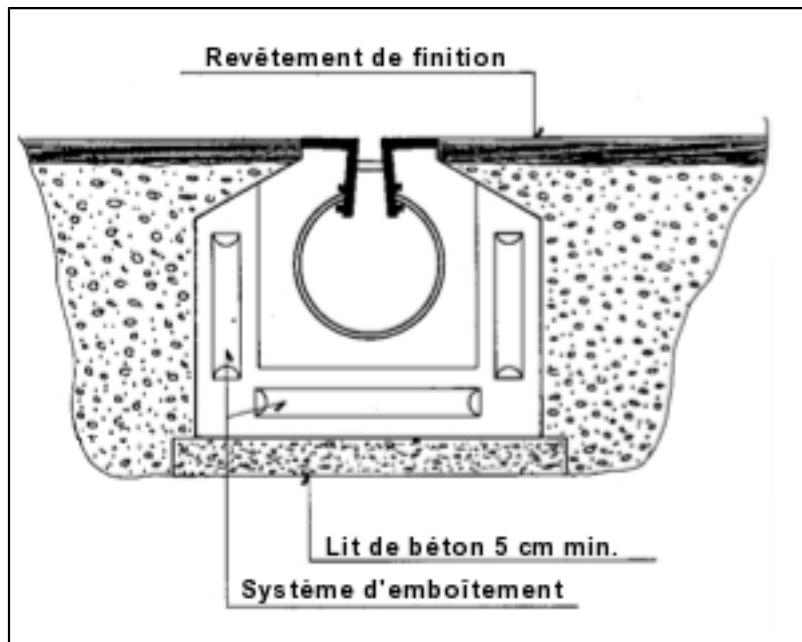
Vue du "SLOT DRAIN"
