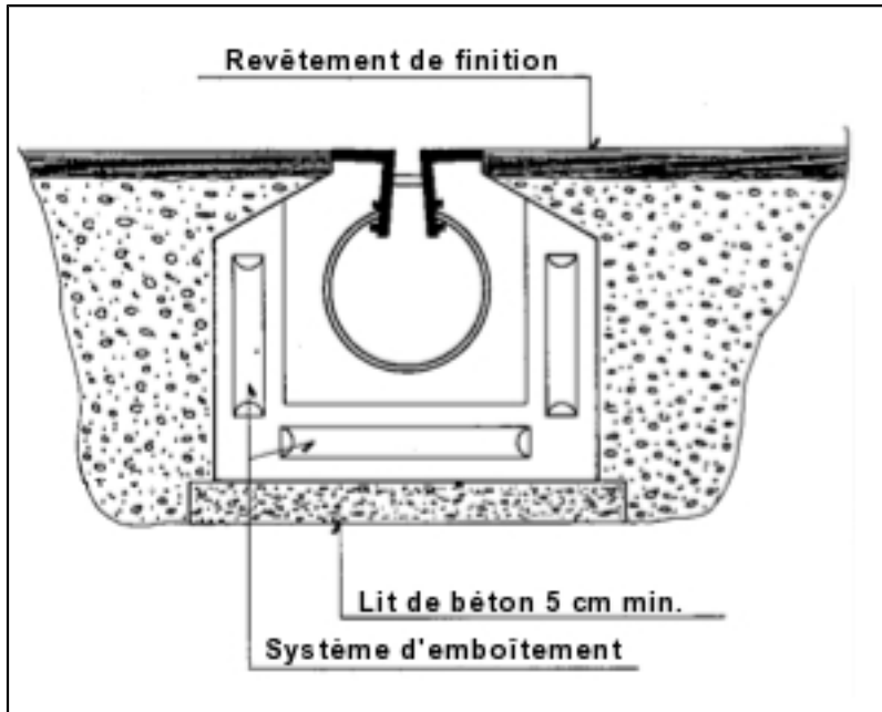
Vue du "SLOT DRAIN"
