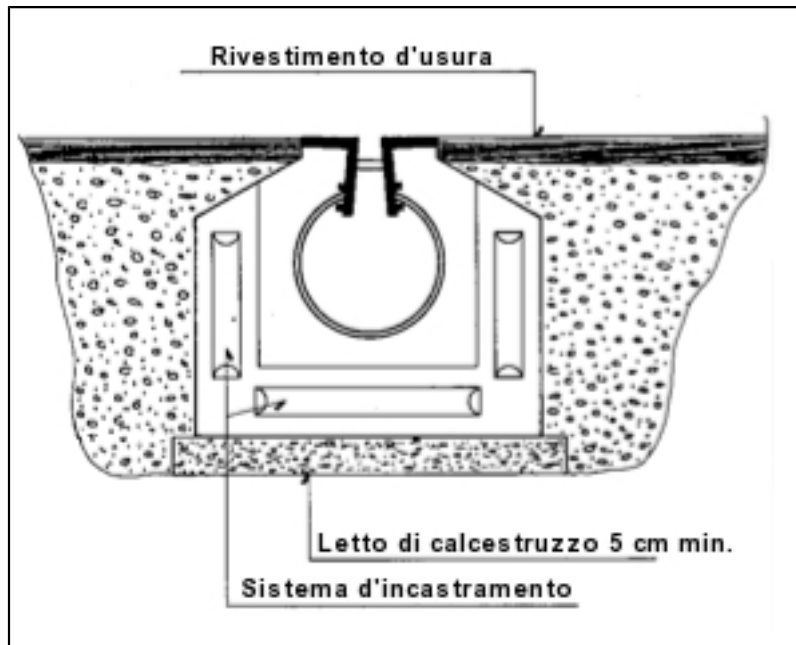
Vista del "SLOT DRAIN"
