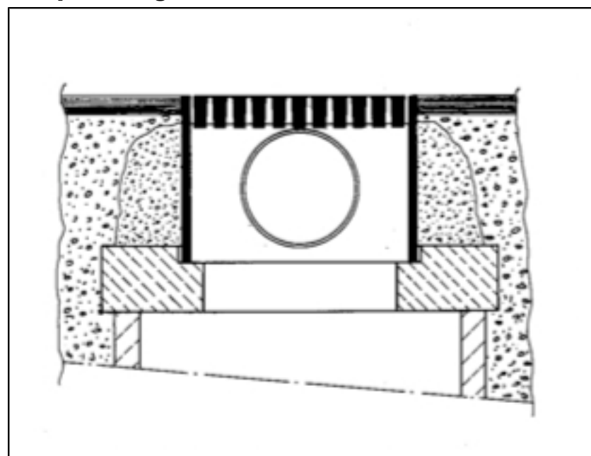
Coupe de la grille
