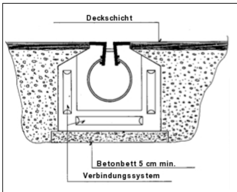
Ansicht "SLOT DRAIN"
